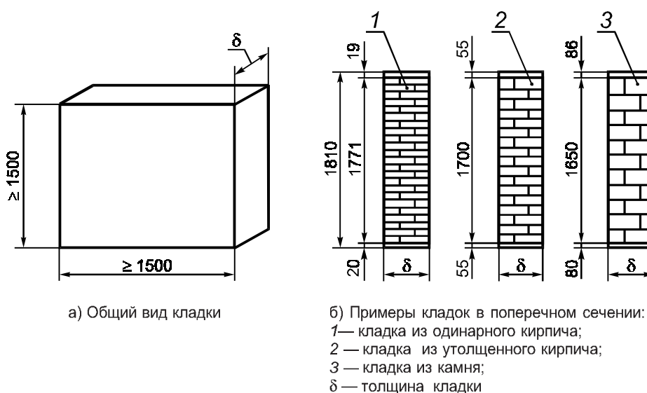
Рисунок 2 — Фрагмент кладки для определения теплопроводности
