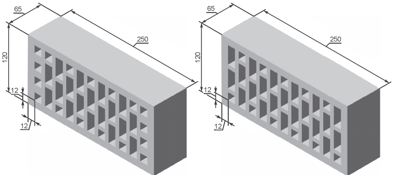
Рисунок А.1.9 — Кирпич формата 1 НФ с 35 пустотами
