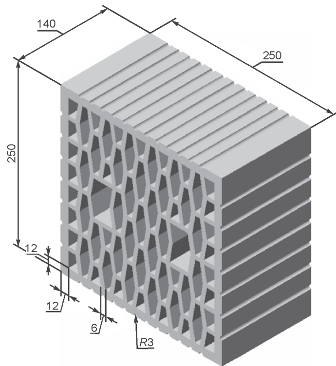
Рисунок А.1.20 — Камень крупноформатный 4,5 НФ
